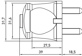
Рис. 1 e.plug.001.10, .plug.002.10
