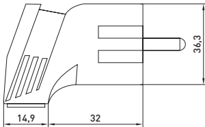
Рис. 3 e.plug.angle.007.16, e.plug.angle.008.16
