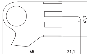
Рис. 4 e.plug.angle.005.16, e.plug.angle.006.16
