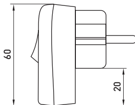
Рис. 5 e.plug.angle.009.16
